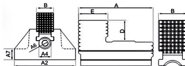
Castanha reversível com 1 degrau - BCR12
