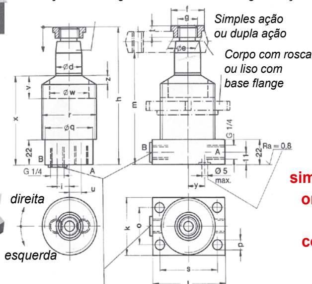
Posição de montagem com Porca KM e Flange Postiço
