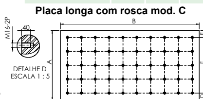
Placa longa com rosca mod. C
