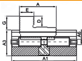
Castanha reversível com 1 degrau - BCR12
