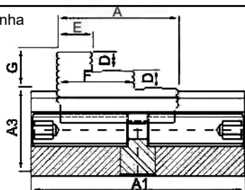
Castanha reversível com 1 degrau - BCR15 - BCR17 - BCR20
