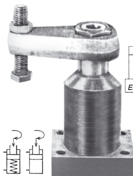
Posição de montagem com Porca KM e Flange Postiço
