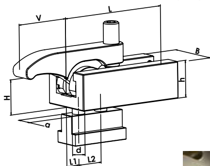
Para Máquina com placa de rosca (TRF)
