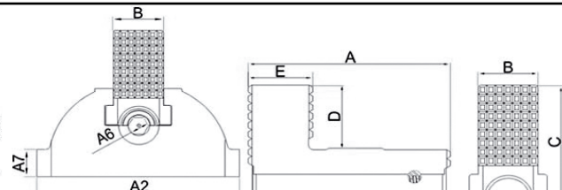
Castanha reversível com 1 degrau - BCR15 - BCR17 - BCR20
