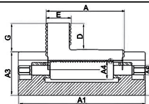
Castanha reversível com 1 degrau - BCR15 - BCR17 - BCR20
