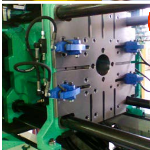
detalhe fixação molde
