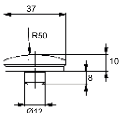
cabeça esférica Ref. 1A Ø 38
