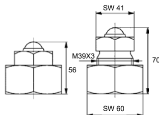
cabeça de ajuste com esfera Ref. 5E SW60
