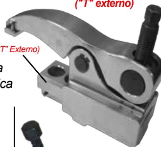
TRU-M12 a M30 ("T" externo)
